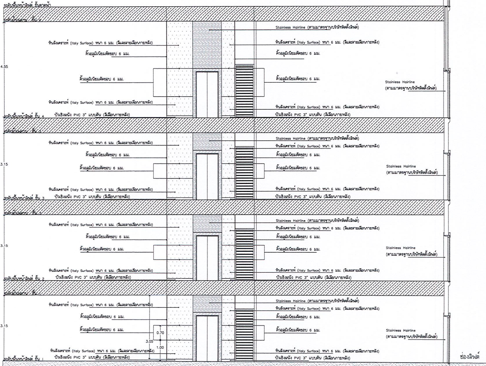
แบบตกแต่งผนังหน้าลิฟต์ มาตราส่วน 1:75
