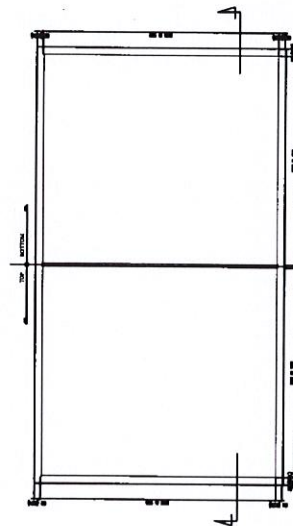
แปลนฐานราก ขนาด 10x3 เมตร
