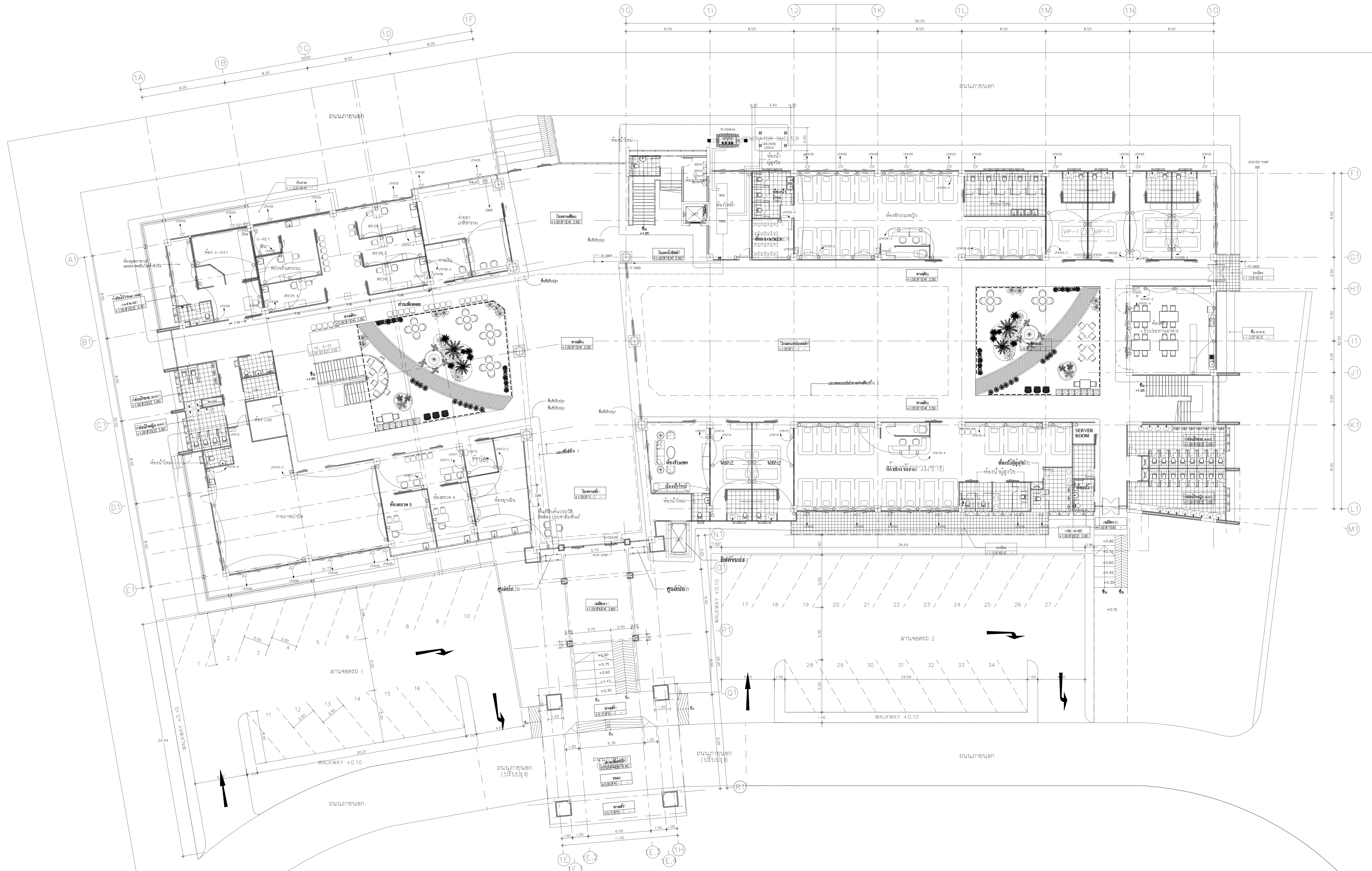
แปลนพื้นชั้น 1 แปลนปรับปรุง 7 กย. 2566
